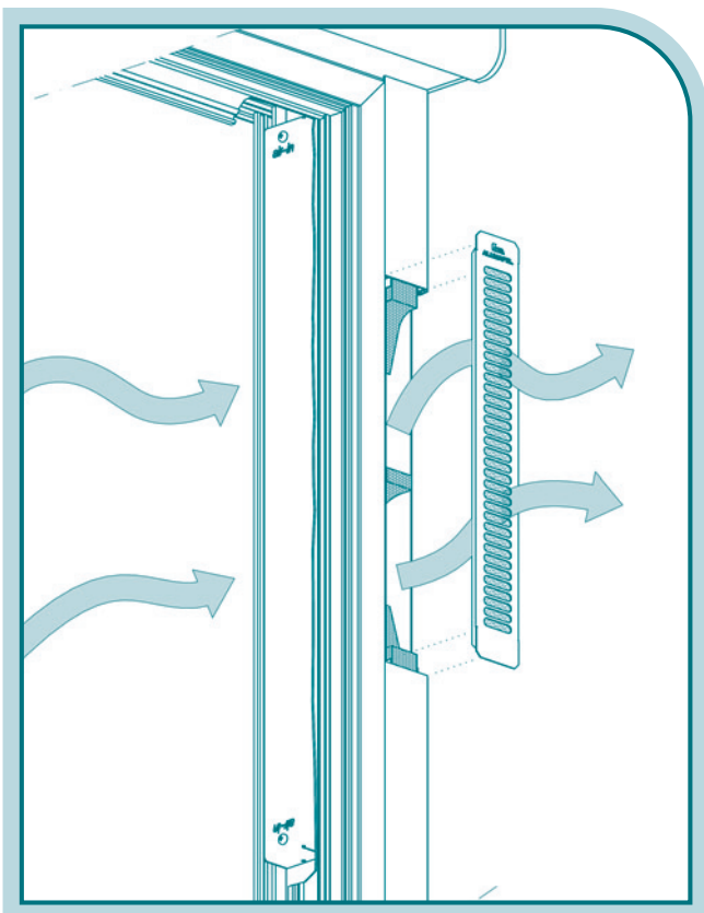
Sistema de aireación ALUMAFEL
