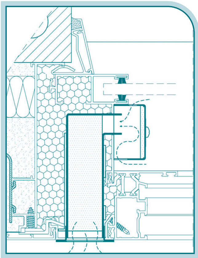
Detalle sección con sistema de aireación alaire
